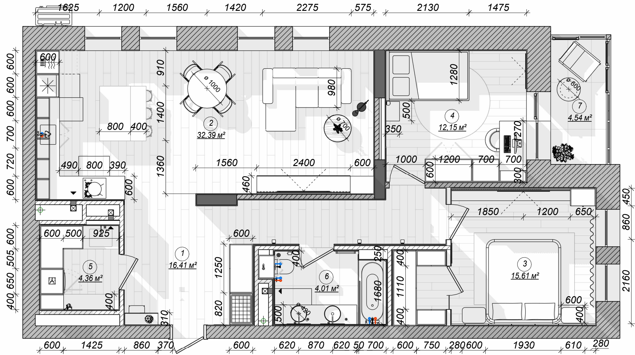
План меблів 1 : 60
