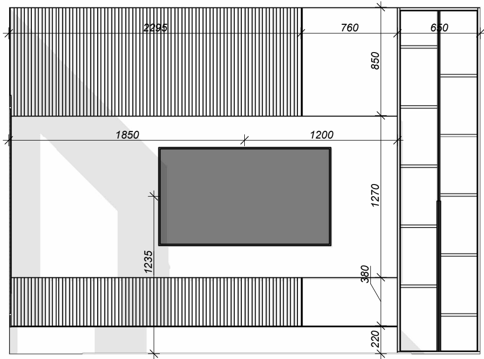
Розгортка 1-а 1 : 30
