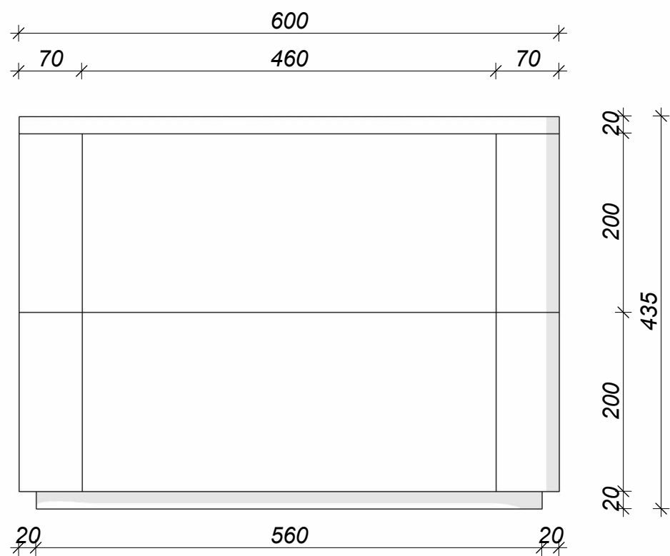
Вигляд спереду 1 : 6
