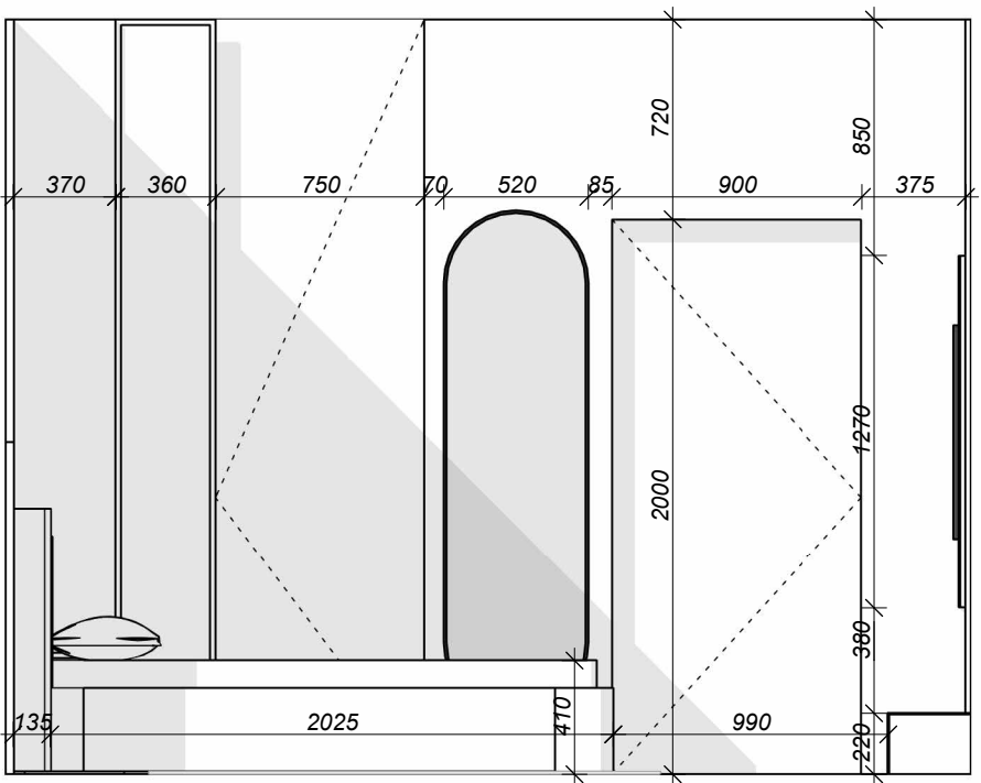
Розгортка 4-г 1 : 30
