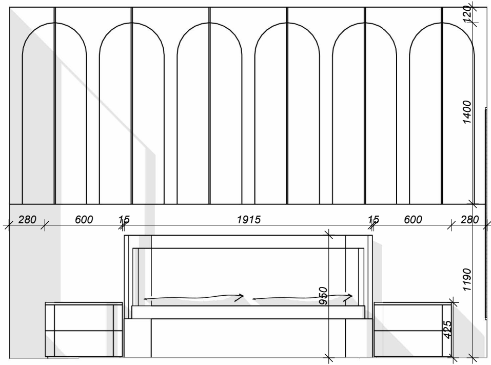
Розгортка 3-в 1 : 30
