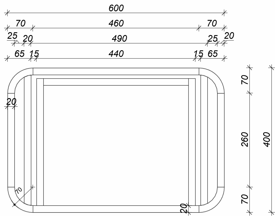
Вигляд зверху 1 : 6
