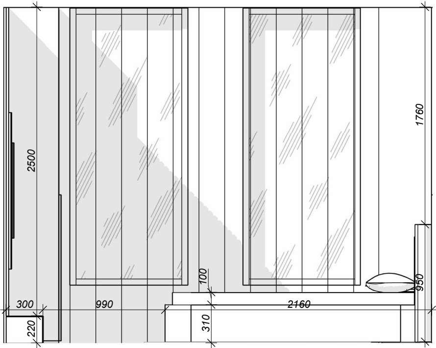
Розгортка 2-б 1 : 30
