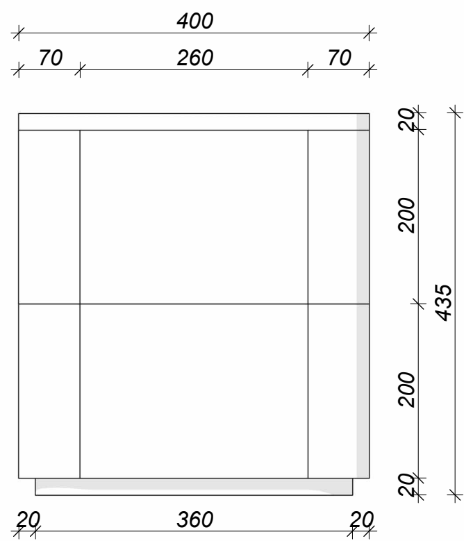
Вигляд збоку 1 : 6
